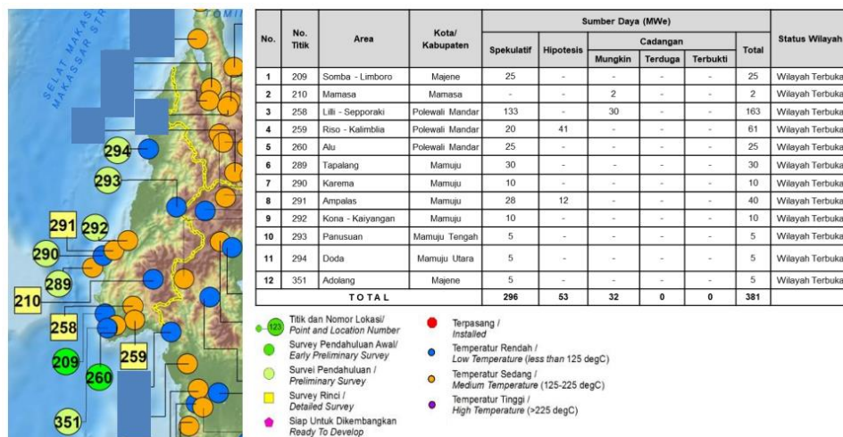
Gambar 2.9 Rincian Potensi Panas Bumi Provinsi Sulawesi Barat
